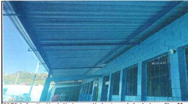
FOTO 6: Sustrucción de lámina, por lámina troquelada aluzinc calibre 26. En aulas.
